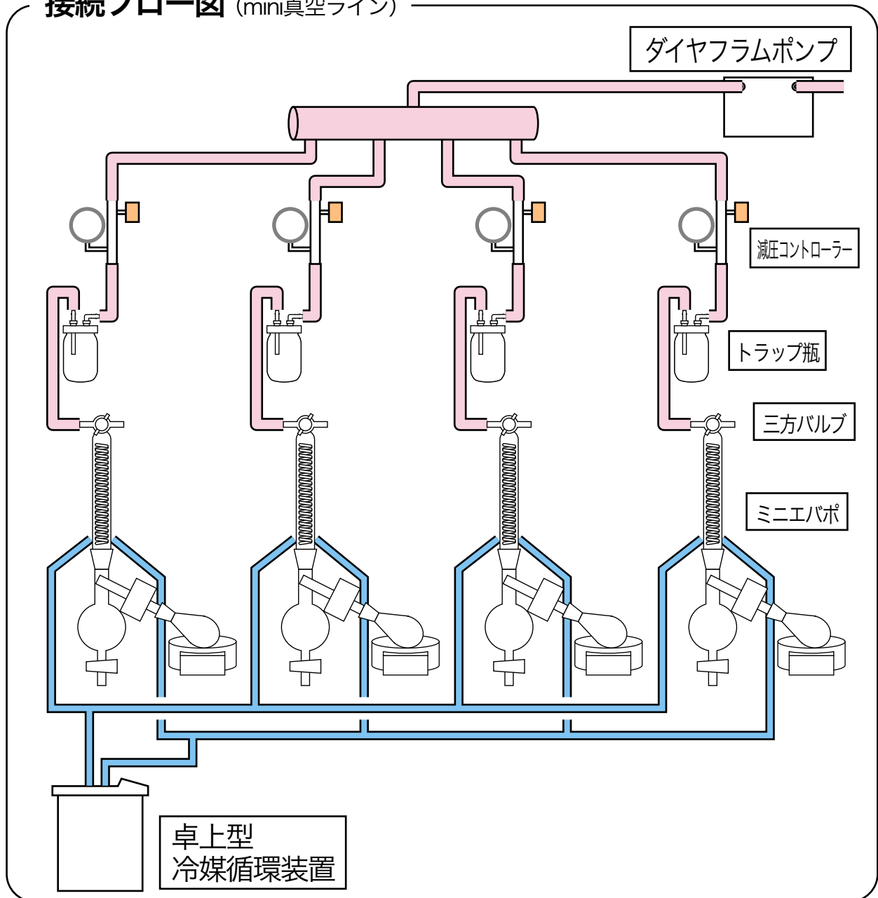
接続フロー図 (mini真空ライン)
